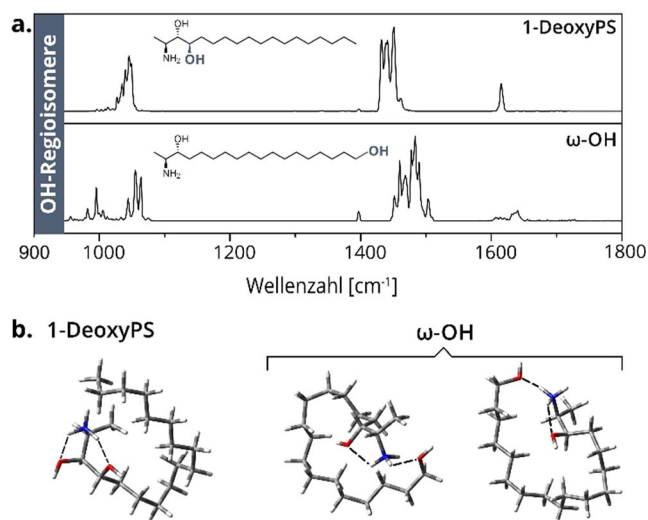
Abbildung 3. IR-Spektren und berechnete Strukturen von OH-Regioisomeren. a) IR-Spektren der OH-Regioisomere 1-DeoxyPS und \omega -OH. Sowohl die Gerüstschwingungen als auch die \text{NH}_3^+ -Biegeschwingungen unterscheiden sich deutlich. b) Energetisch günstige Konformere von 1-DeoxyPS und \omega -OH. Die gleichzeitige Koordination der \text{NH}_3^+ -Gruppe an beide Hydroxylgruppen wird für beide Isomere beobachtet. Im Fall von \omega -OH koexistieren mehrere Konformere.
