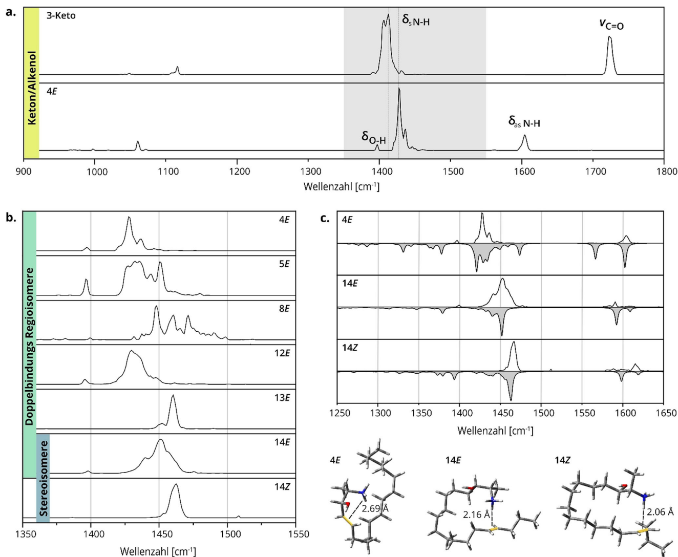
Abbildung 2. Gasphasen-IR-Spektren und Niedrigenergie-Strukturen von 1-Deoxysphingolipiden. a) IR-Spektren der Isomere 3-Keto und 4E. Das Keton und Alkenol sind anhand diagnostischer Streckenschwingungen ( \nu ) und Biegeschwingungen ( \delta ) unterscheidbar. Die intensivste Bande in dem grau unterlegten Bereich wird durch die \text{NH}_3^+ -umbrella-Mode verursacht. b) Gestapelte IR-Spektren von 1-DeoxySO-C=C-Regio- und Stereoisomeren in der Region der \text{NH}_3^+ -umbrella-Schwingung ( 1350\text{--}1550\text{ cm}^{-1} ). Die Absorptionsmuster und Schwingungsfrequenzen hängen von der C=C-Position und -Konfiguration ab. c) Spektrale Übereinstimmung mit berechneten IR-Spektren (grau) von DFT-optimierten Strukturen von 4E, 14E und 14Z im Bereich der \text{NH}_3^+ -Biegeschwingungen. Die zugehörigen theoretischen Strukturen verdeutlichen die unterschiedlichen Geometrien der Ladungs-Olefin-Interaktionen.
